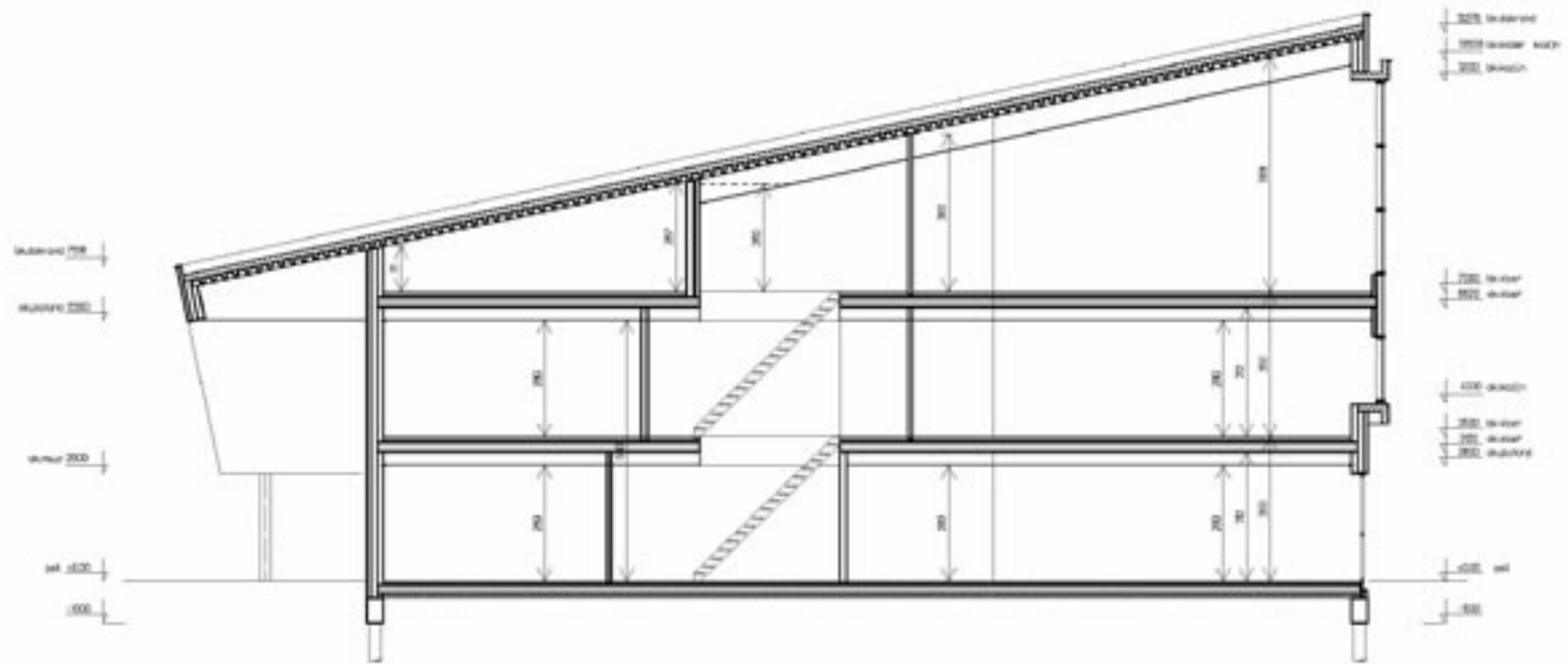
DOORSNEDE E-E
