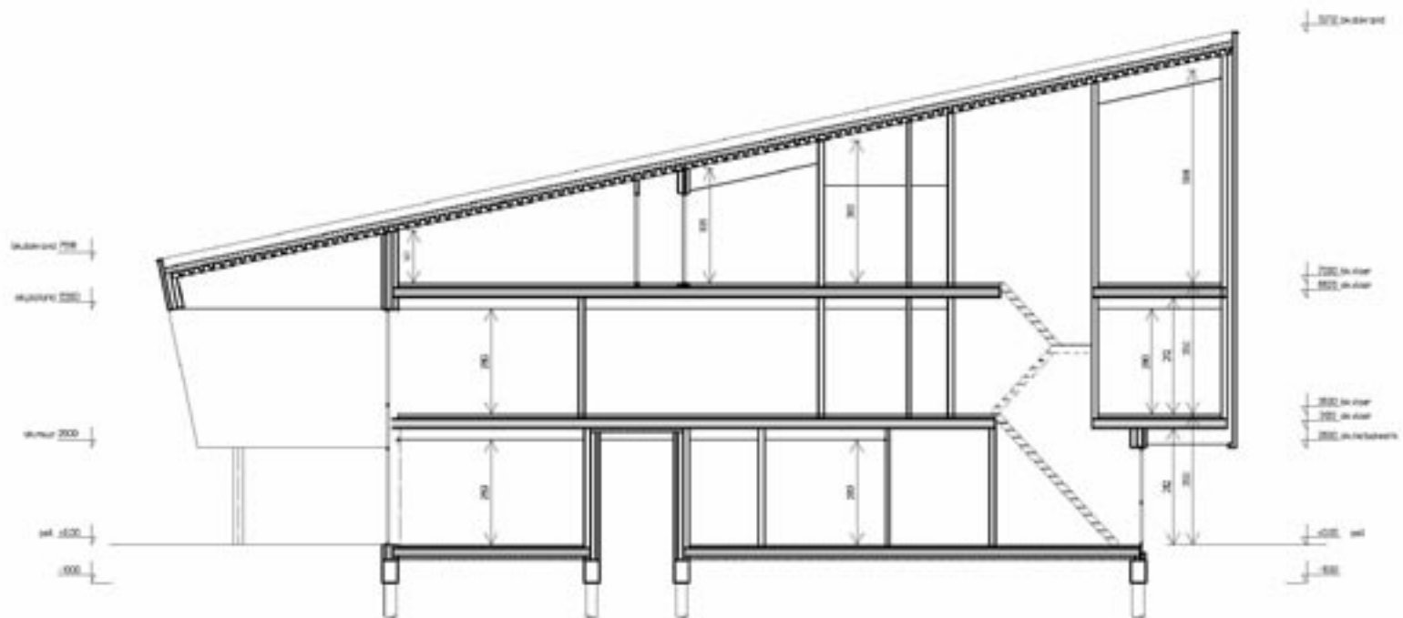
DOORSNEDE D-D
